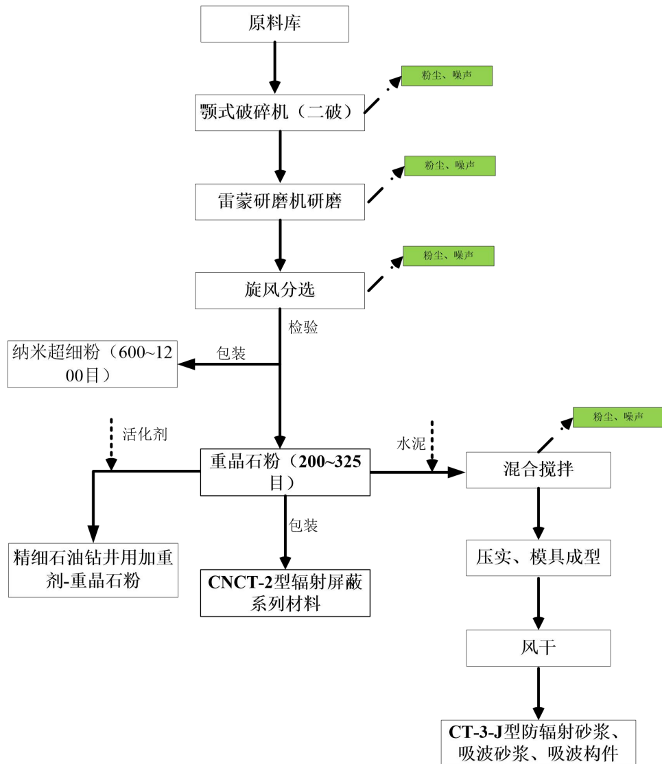
图 2-4 重晶石矿生产工艺流程及产污环节图
