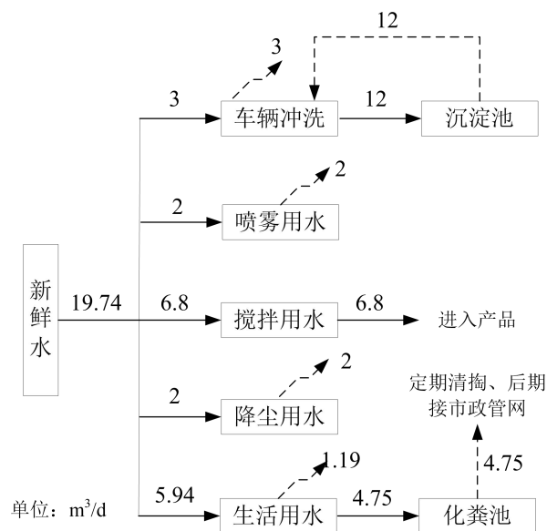
图 2-1 本项目水平衡图
